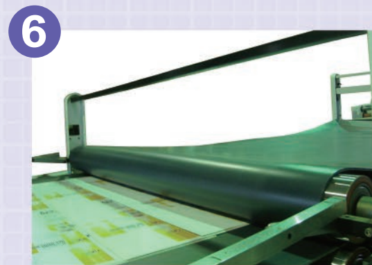
6 加壓輸送機 Pressurized Delivery
